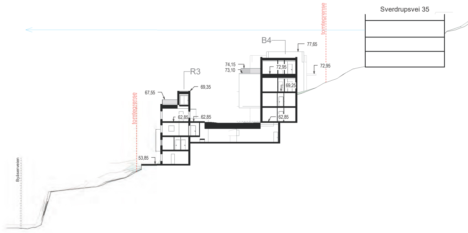
Tverrsnitt B4-R3
