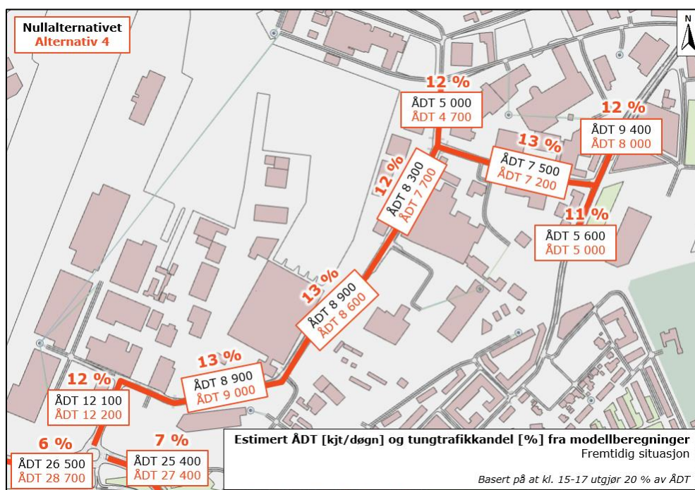
Figur 5-39: Anslått ÅDT [kjt/døgn] og tungtrafikkandel [%] gjennom Nyhavna i prognoseår 2035, nullalternativet og alternativ 4 OBS: det gjøres oppmerksom på at bakgrunnskartet kun viser geometrien til alternativ 4.
