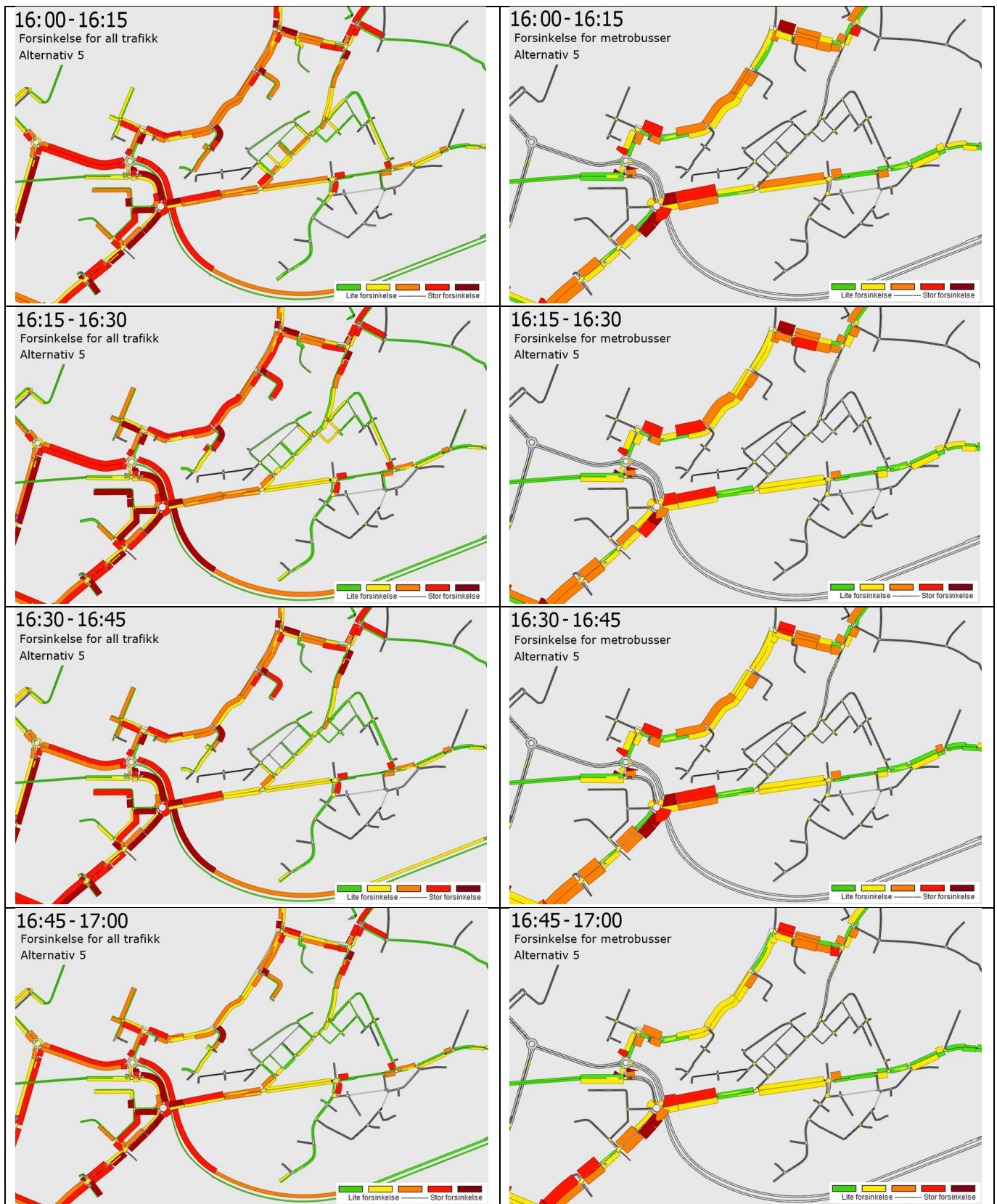
Figur 5-35: Forsinkelsesplot per kvarter i alternativ 5, ettermiddag. All trafikk er vist til venstre og metrobuss til høyre.
