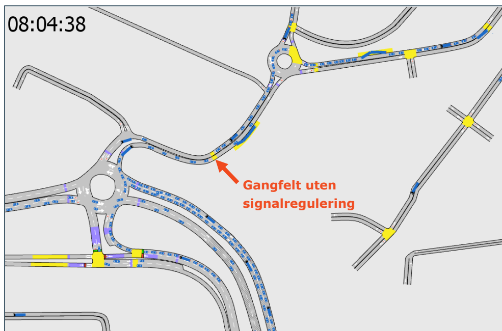
Figur 7-26: Uttak fra simulering viser køoppbygging foran angitt gangfelt som gir konsekvenser for trafikken ut av Strindheimtunnelen
