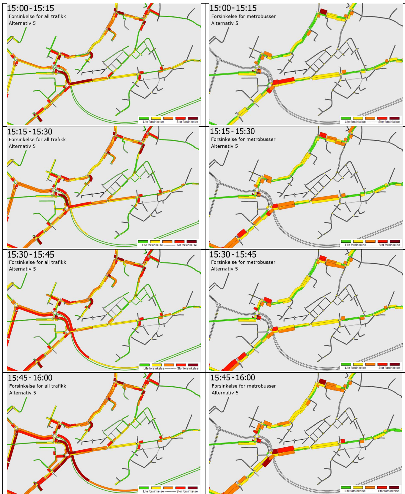
Figur 5-35 viser forsinkelsesplot per kvarter for alternativ 5 om ettermiddagen; for all trafikk i venstre kolonne, og for kun metrobusser i høyre kolonne.
