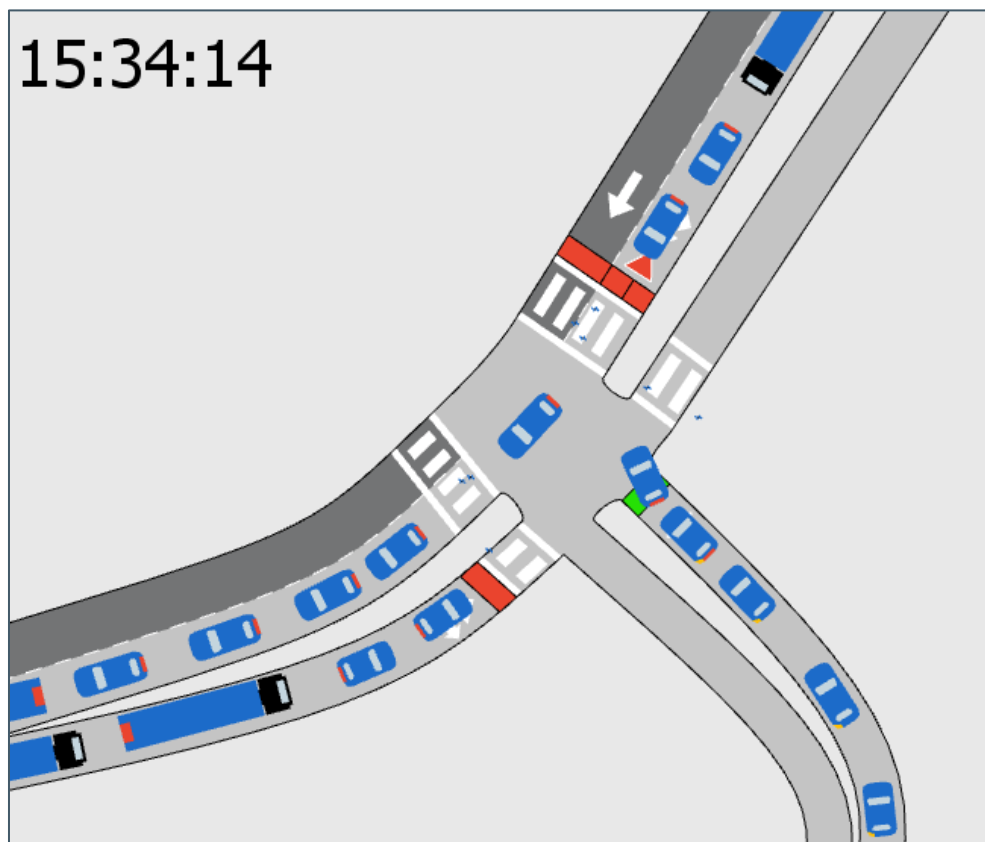
Figur 5-32: Simulering viser køoppbygging i alt. 4 ut fra Strandveien pga. kø i Maskinistgata og konflikt med gangfelt som har grønt signal samtidig som trafikken fra Strandveien.
