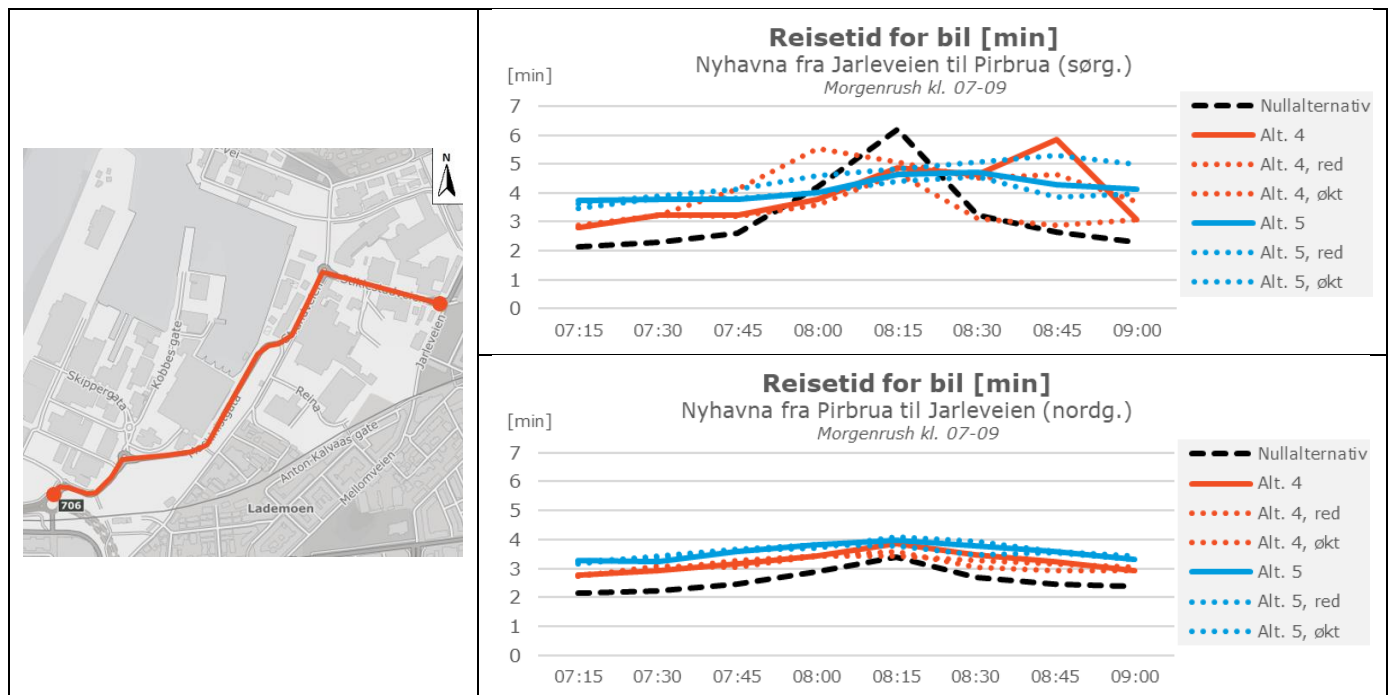
Figur 5-19: Reisetid for biltrafikken gjennom Nyhavna, følsomhetsberegninger med redusert (red) og økt (økt) trafikk, morgen
