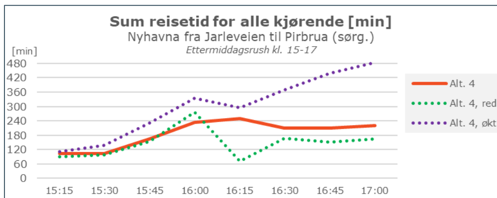
Figur 5-38: Sum reisetid for alle kjørende gjennom Nyhavna i sørgående retning, følsomhetsberegninger med redusert og økt trafikk, ettermiddag
