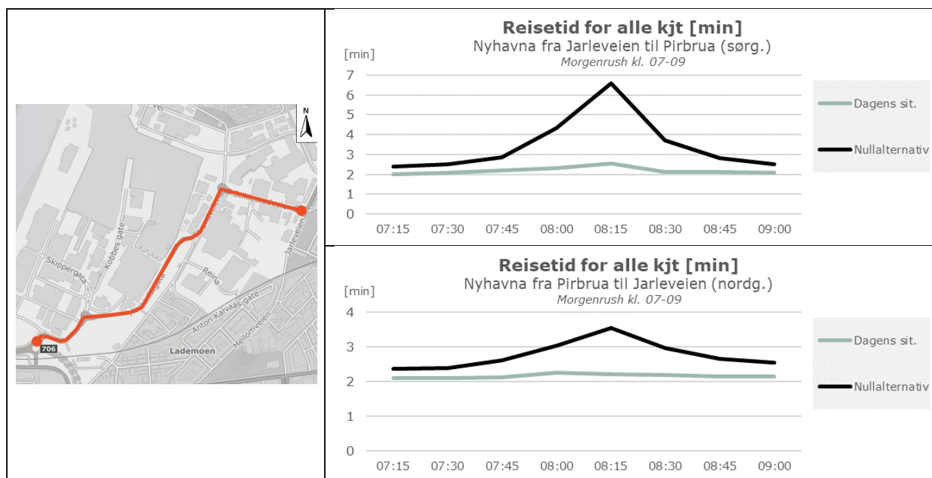
Figur 5-2: Reisetid for alle kjørt gjennom Nyhavna, dagens og nullalternativet, morgen
