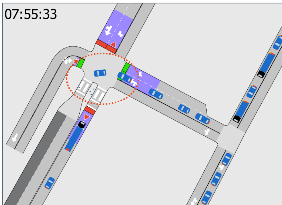
Figur 7-31: Simulering av kjørende fra Strandveien som må vente på kryssende over gangfeltet i Maskinistgata
