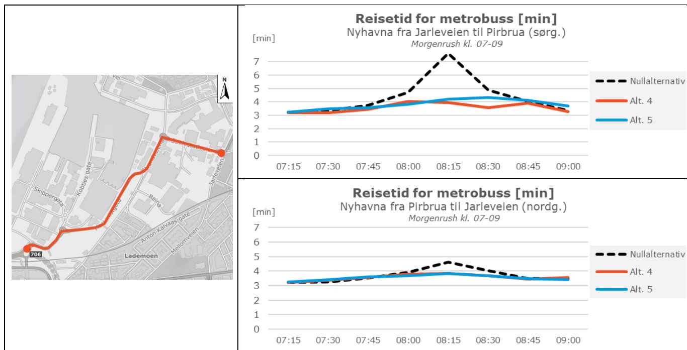
Figur 5-3: Reisetid for metrobusser gjennom Nyhavna, morgen
