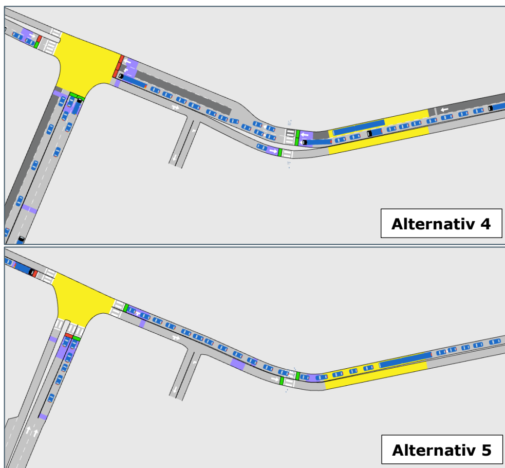
Figur 6-1: Buss blir stående langt bak på holdeplass ved kø i Maskinistgata i alt. 5
