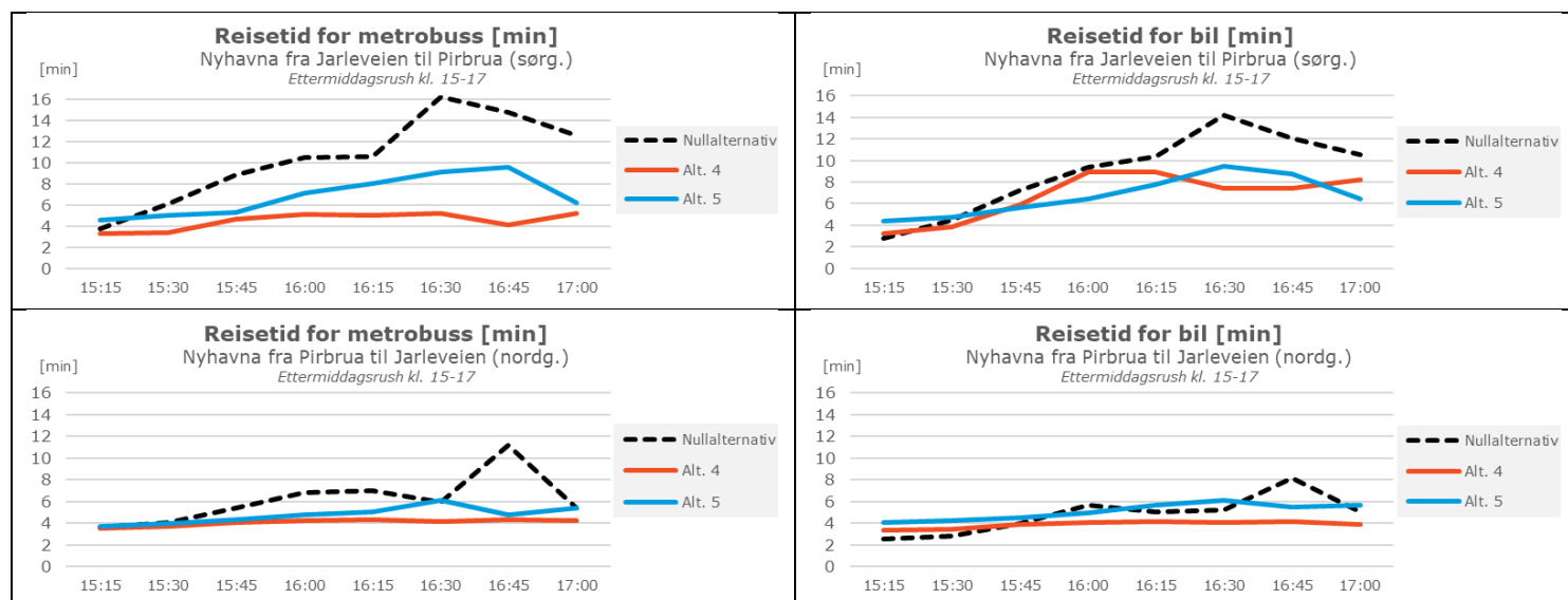
Figur 5-29: Reisetid gjennom Nyhavna for metrobusser (t.v.) og biler (t.h.), ettermiddag
