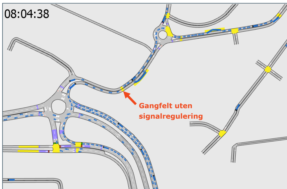
Figur 5-5: Uttak fra simulering av nullalternativet viser køoppbygging foran angitt gangfelt som gir konsekvenser for trafikken ut av Strindheimtunnelen
