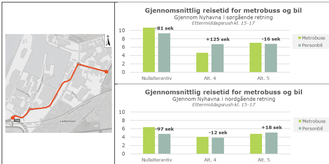
Figur 5-30: Gjennomsnittlig reisetid gjennom Nyhavna, ettermiddag
