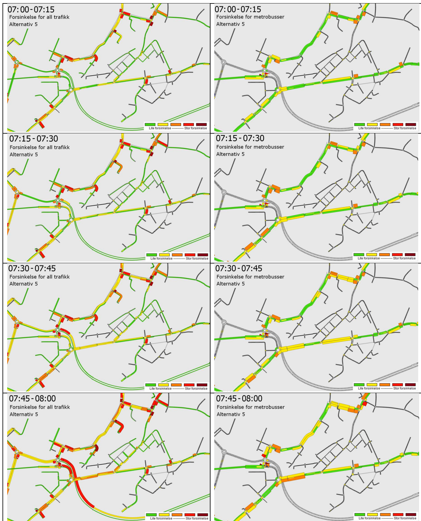
Figur 5-17 viser forsinkelsesplot per kvarter for alternativ 5 om morgenen; for all trafikk i venstre kolonne, og for kun metrobusser i høyre kolonne.
