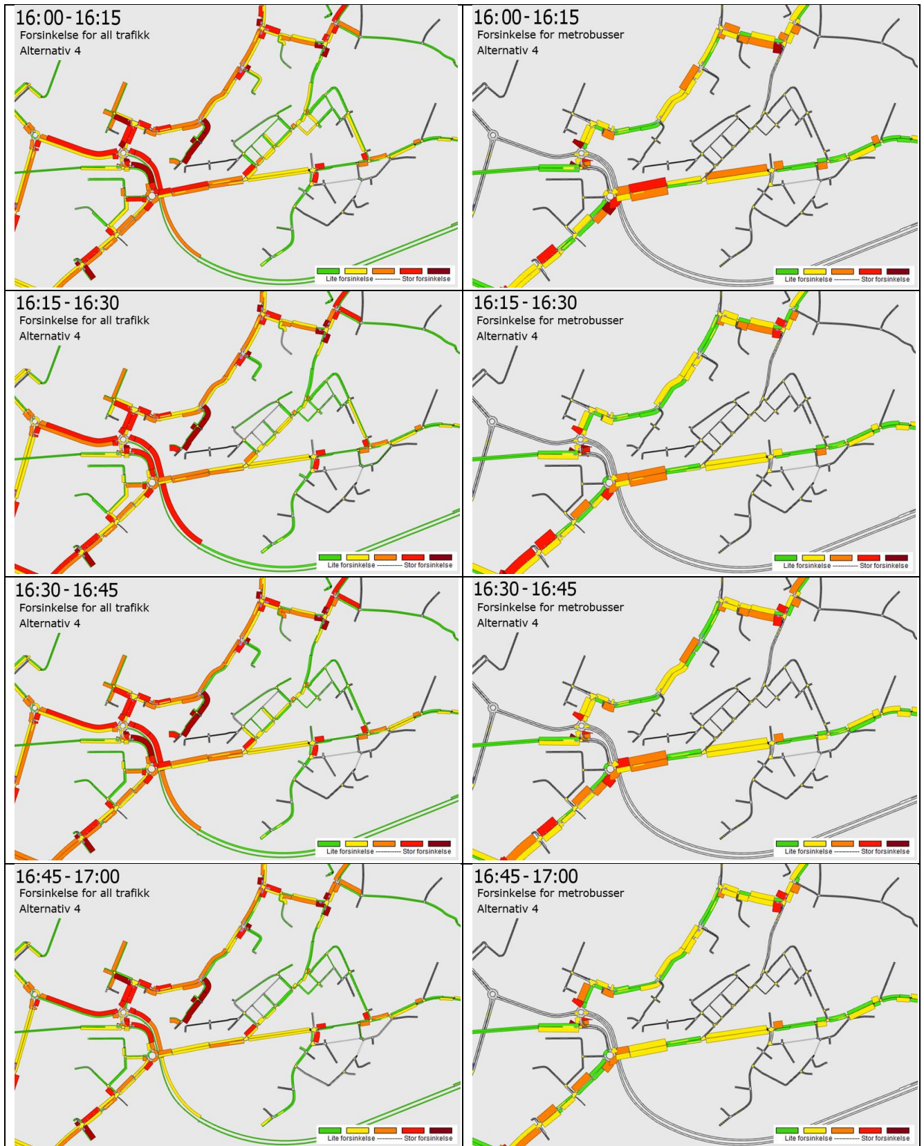
Figur 5-34: Forsinkelsesplot per kvarter i alternativ 4, ettermiddag. All trafikk er vist til venstre og metrobuss til høyre.
