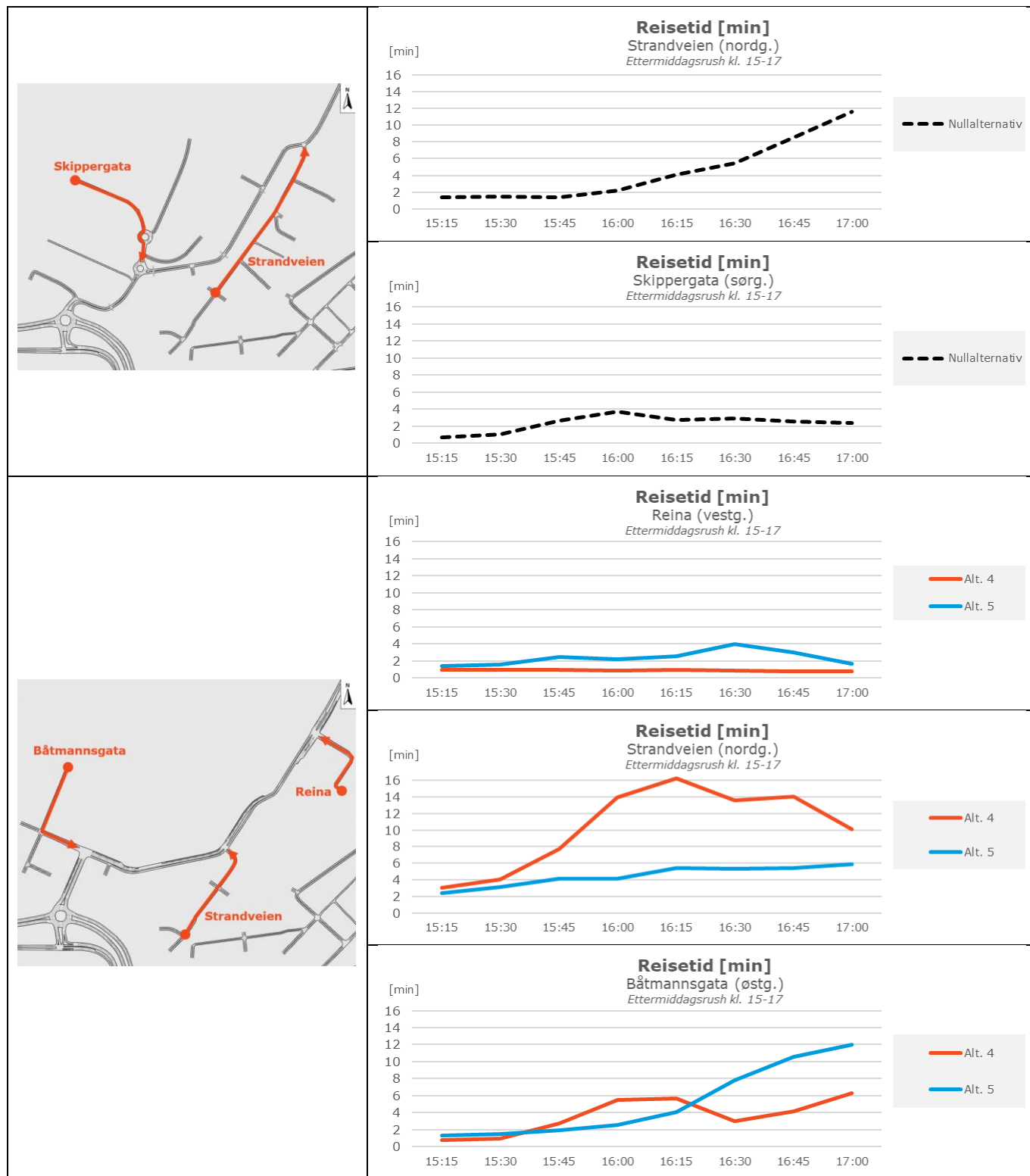
Figur 5-31: Reisetid for kjørende ut fra utbyggingsområder, ettermiddagen
