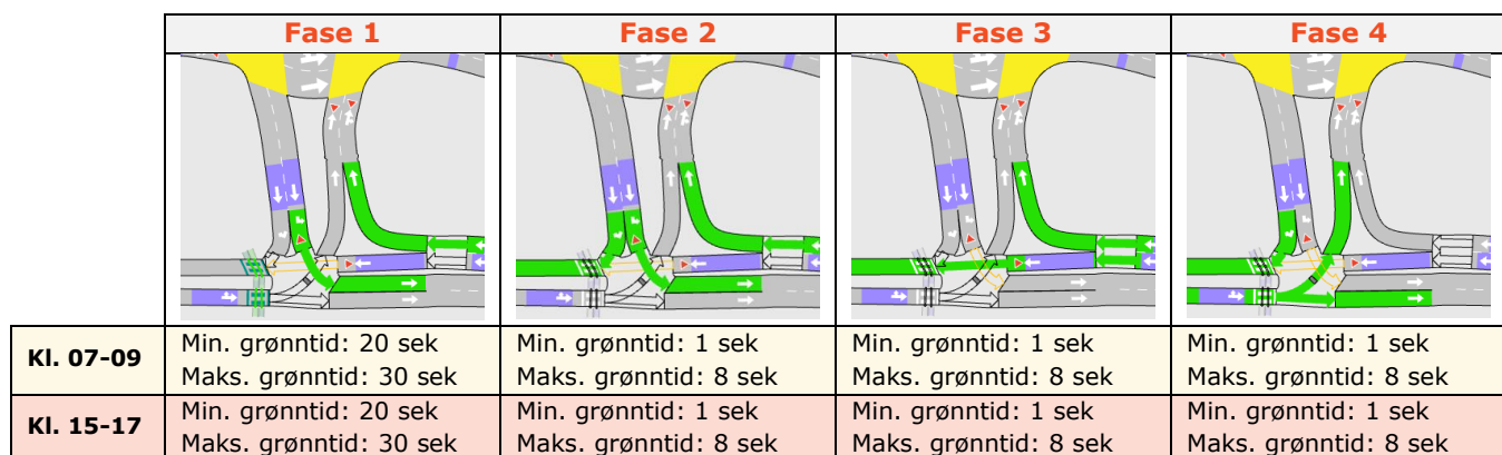
Figur 4-12: Kodet signalplan i kryss mellom Dyrø Halses gate og Nidelv bru i alt. 4
