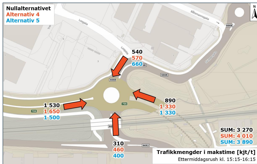
Figur 5-27: Sammenligning av avviklet trafikk [kjt/t] nullalternativet, alt. 4, og alt. 5 i rundkjøring ved Strindheimtunnelen, ettermiddag
