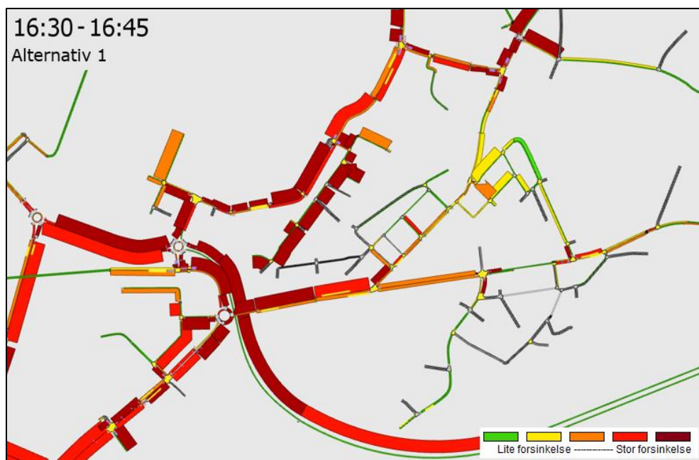
Figur 7-39: Forsinkelsesplot for det mest belastede kvarter om ettermiddagen, alt. 1
