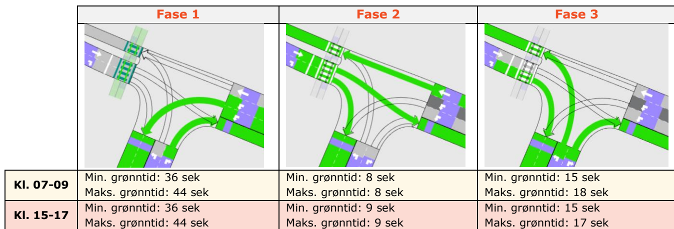
Figur 4-11: Kodet signalplan i kryss mellom Maskinistgata og Skippergata i alt. 4
