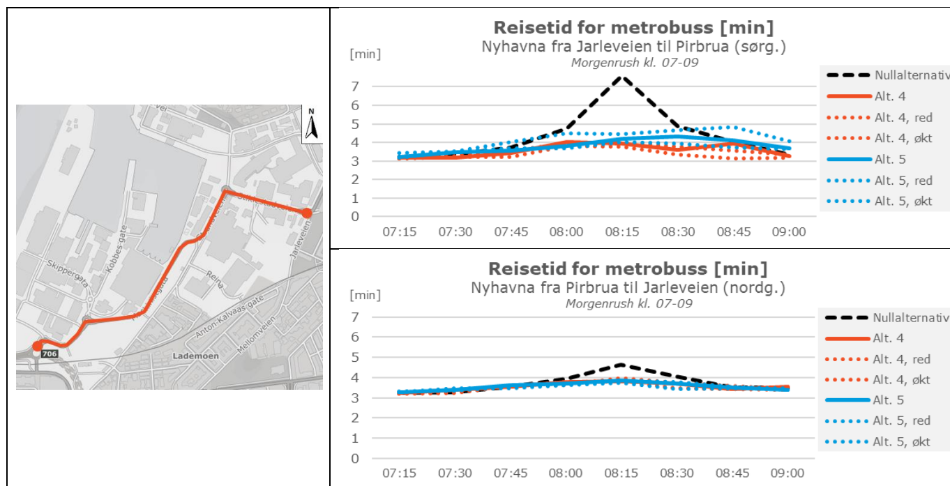
Figur 5-18: Reisetid for metrobusser gjennom Nyhavna, følsomhetsberegninger med redusert (red) og økt (økt) trafikk, morgen
