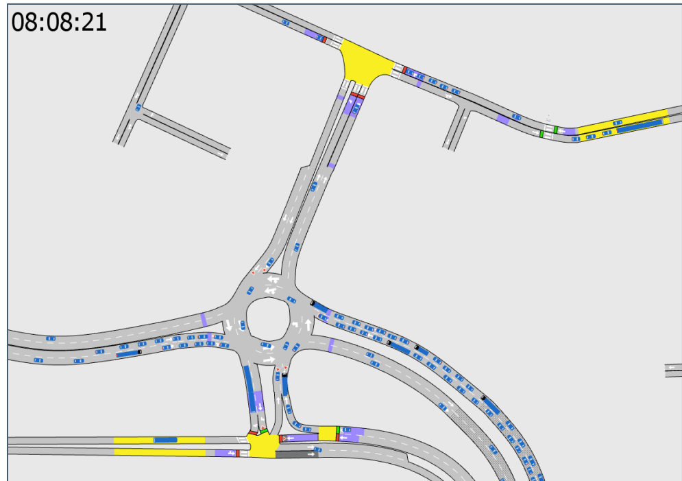
Figur 5-6: Uttak fra simulering av alternativ 5 ved rundkjøringen med Strindheimtunnelen
