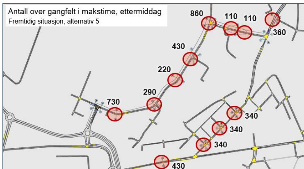
Figur 3-13: Antall over gangfelt i Aimsun makstime ettermiddag, alt. 5
