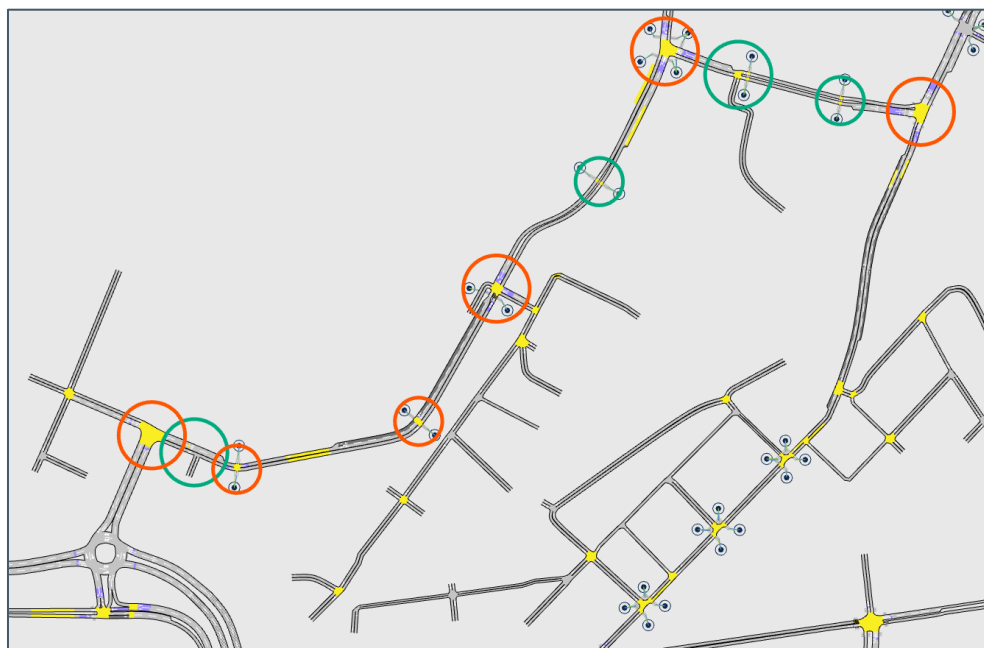
Figur 7-11: Signalregulerte og vikepliktregulerte kryss gjennom Nyhavna i alt. 1
