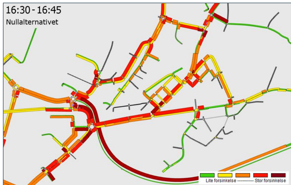
Figur 5-24: Forsinkelsesplot for det mest belastede kvarter om ettermiddagen, nullalternativet
