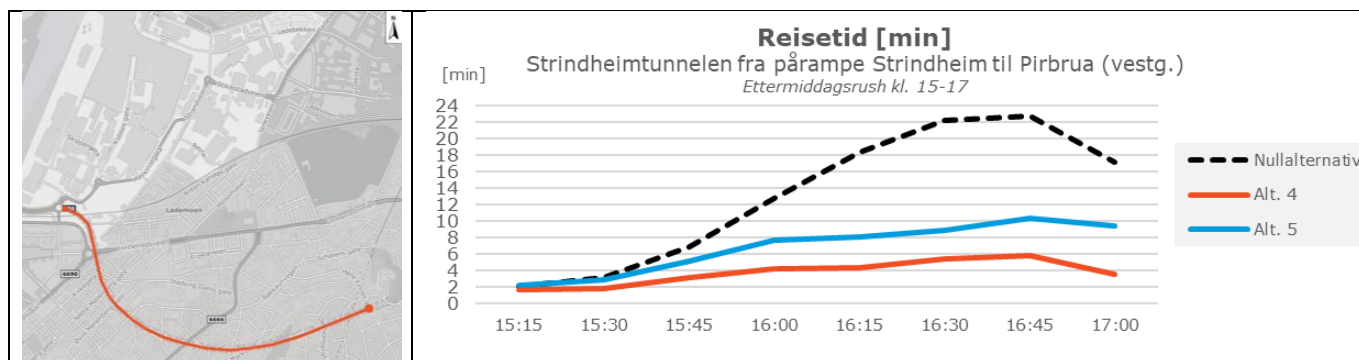
Figur 5-22: Reisetid i Strindheimtunnelen i vestgående retning, ettermiddag
