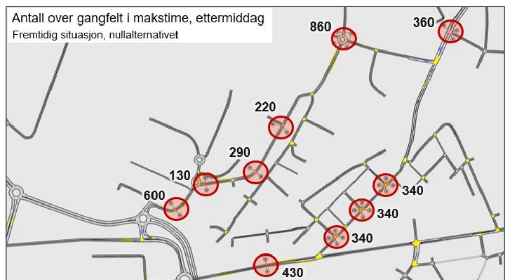
Figur 3-11: Antall over gangfelt i Aimsun i makstime ettermiddag, nullalternativet
