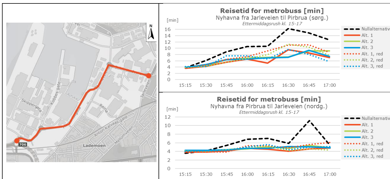
Figur 7-46: Reisetid for metrobusser gjennom Nyhavna, følsomhetsberegninger med redusert trafikk, ettermiddag
