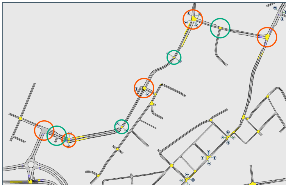
Figur 7-2: Signalregulerte og vikepliktregulerte kryss gjennom Nyhavna i alt. 1A
