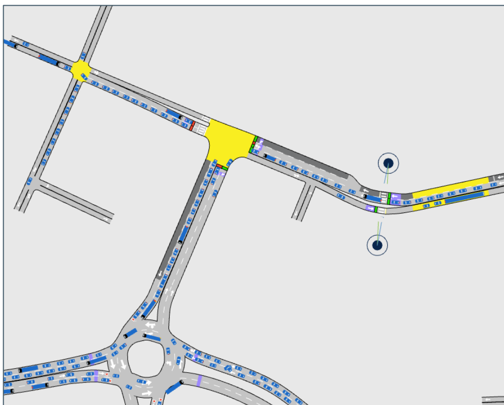
Figur 5-33: Simulering viser kjøppbygging ut fra Båtmannsgata i alt. 4. Trafikk fra Båtmannsgata klarer ikke alltid å kjøre gjennom krysset med Skippergata
