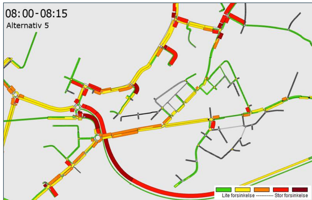
Figur 5-10: Forsinkelsesplot for det mest belastede kvarter om morgenen, alt. 5
