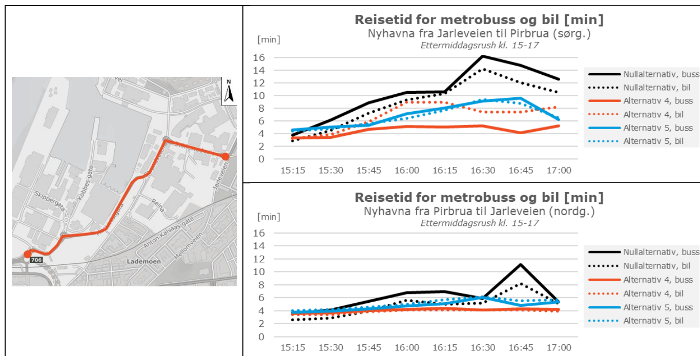
Figur 5-28: Reisetid gjennom Nyhavna for metrobusser og biler, ettermiddag
