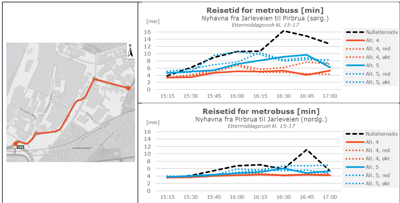
Figur 5-36: Reisetid for metrobusser gjennom Nyhavna, følsomhetsberegninger med redusert (red) og økt (økt) trafikk, ettermiddag
