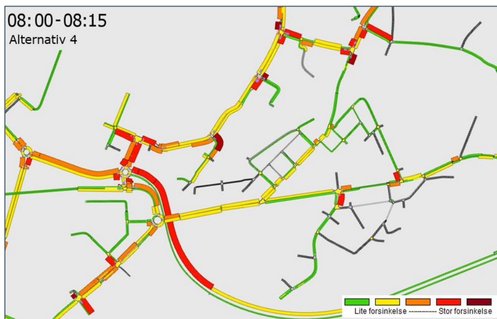
Figur 5-9: Forsinkelsesplot for det mest belastede kvarter om morgenen, alt. 4
