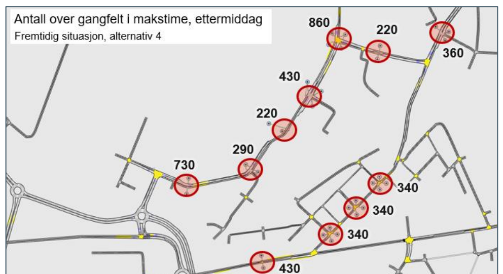
Figur 3-12: Antall over gangfelt i Aimsun makstime ettermiddag, alt. 4
