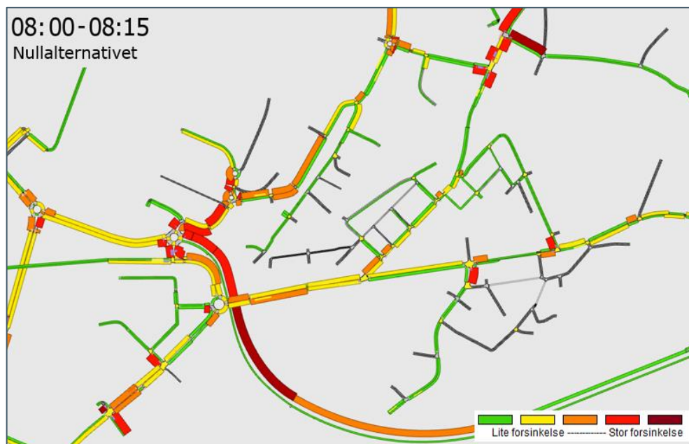
Figur 5-8: Forsinkelsesplot for det mest belastede kvarter om morgenen, nullalternativet
