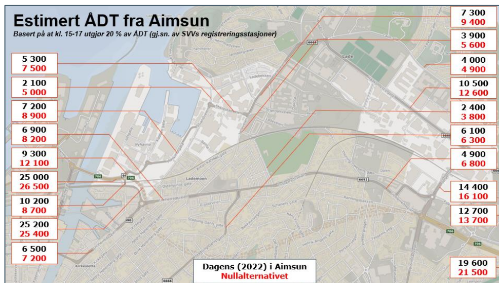
Figur 5-1: ÅDT-estimat for relevante veger i dagens og fremtidig situasjon basert på en forenkling om at trafikkmengder kl. 15-17 utgjør 20 % av ÅDT
