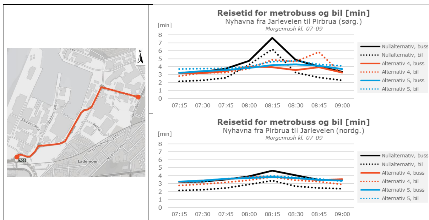
Figur 5-12: Reisetid gjennom Nyhavna for metrobusser og biler, morgen
