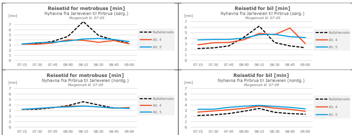
Figur 5-13: Reisetid gjennom Nyhavna for metrobusser (t.v.) og biler (t.h.), morgen
