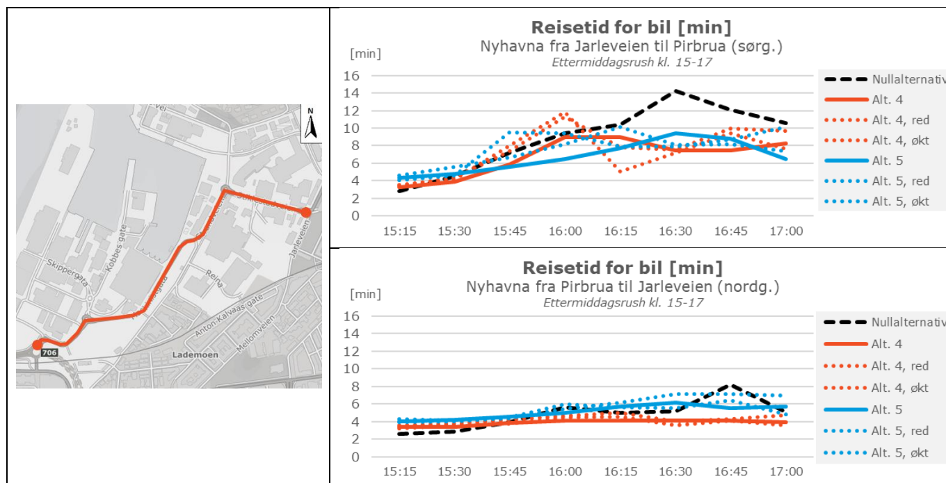
Figur 5-37: Reisetid for biltrafikken gjennom Nyhavna, følsomhetsberegninger med redusert (red) og økt (økt) trafikk, ettermiddag
