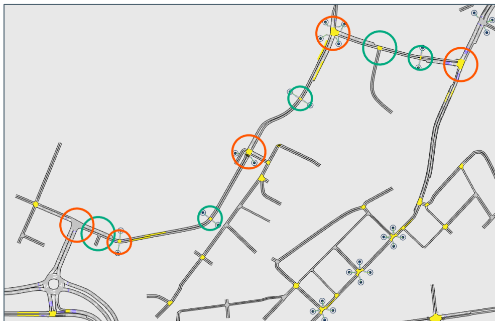
Figur 7-9: Signalregulerte og vikepliktregulerte kryss gjennom Nyhavna i alt. 1A
