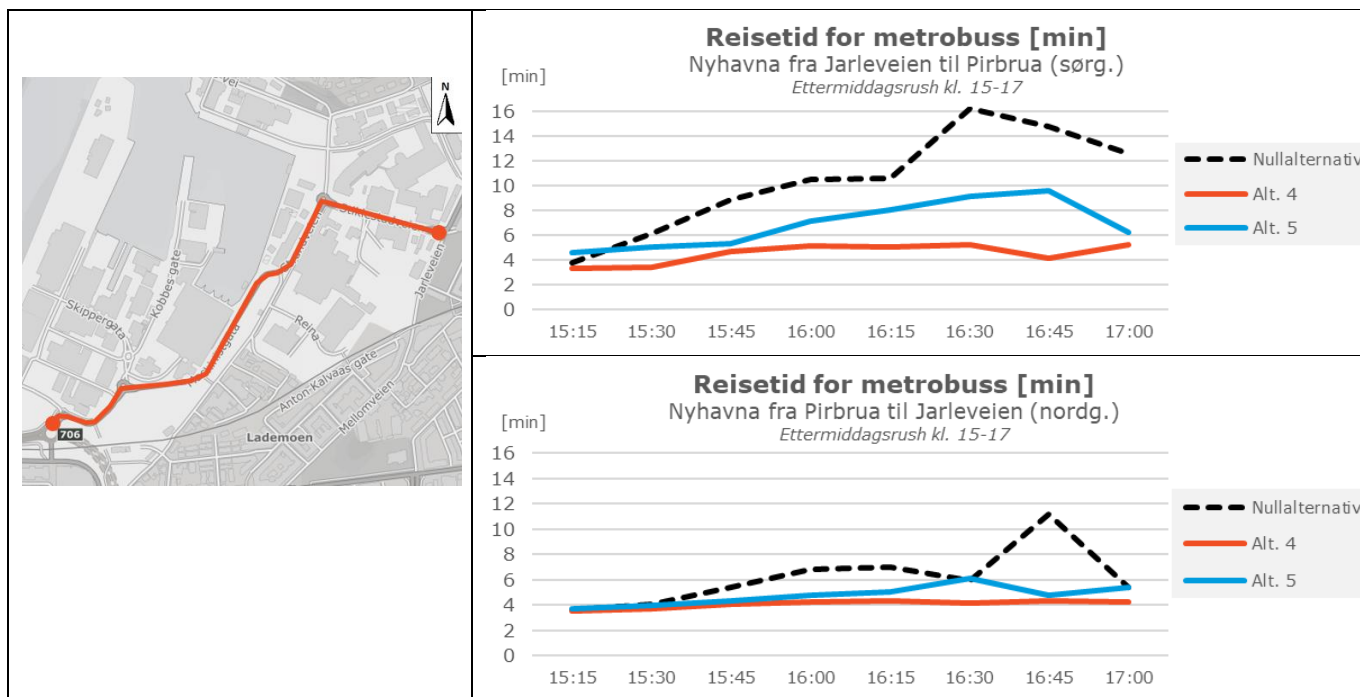
Figur 5-21: Reisetid for metrobusser gjennom Nyhavna, ettermiddag
