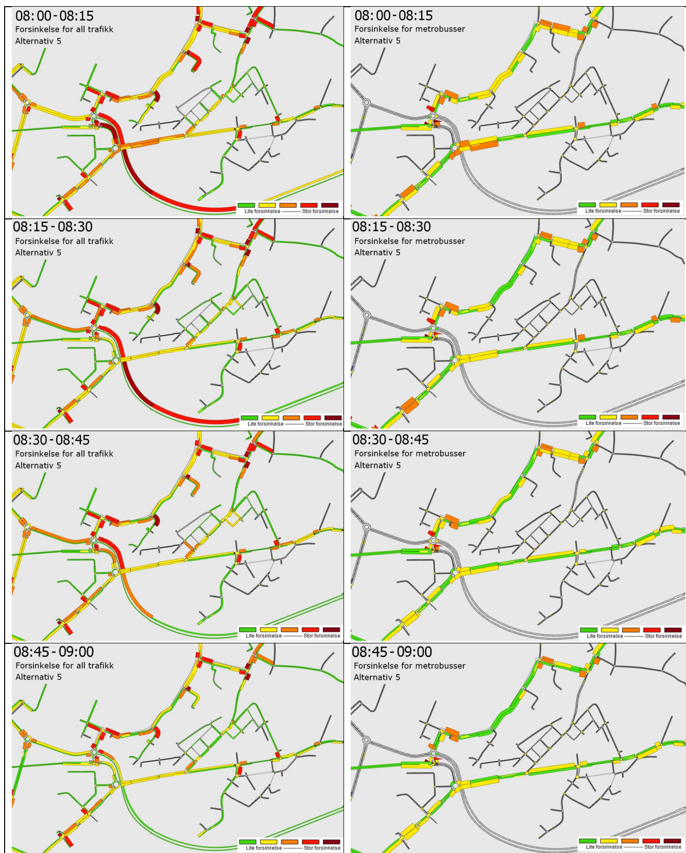
Figur 5-17: Forsinkelsesplot per kvarter i alternativ 5, morgen. All trafikk er vist til venstre og metrobuss til høyre.
