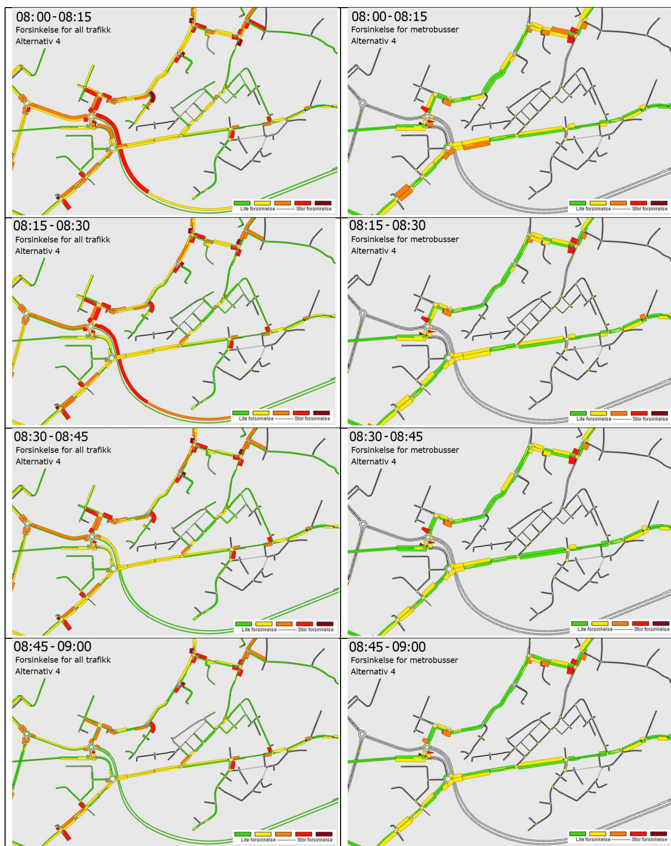
Figur 5-16: Forsinkelsesplot per kvarter i alternativ 4, morgen. All trafikk er vist til venstre og metrobuss til høyre.
