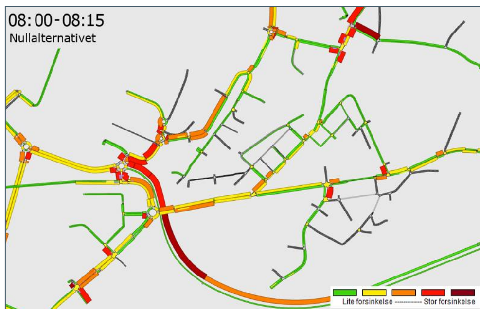
Figur 5-7: Forsinkelsesplot for det mest belastede kvarter om morgenen, nullalternativet
