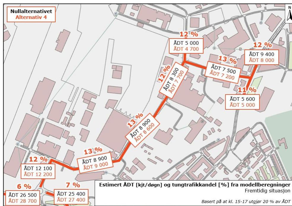
Figur 5-32: Anslått ÅDT [kjt/døgn] og tungtrafikkandel [%] gjennom Nyhavna i prognoseår 2035, nullalternativet og alternativ 4
