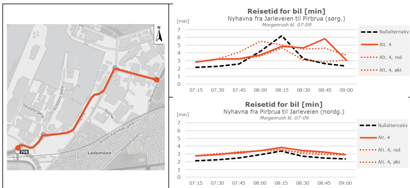
Figur 5-15: Reisetid for biltrafikken gjennom Nyhavna, følsomhetsberegninger med redusert (red) og økt (økt) trafikk, morgen
