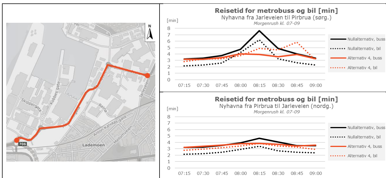
Figur 5-10: Reisetid gjennom Nyhavna for metrobusser og biler, morgen
