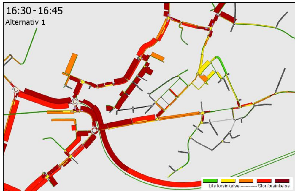
Figur 7-39: Forsinkelsesplot for det mest belastede kvarter om ettermiddagen, alt. 1
