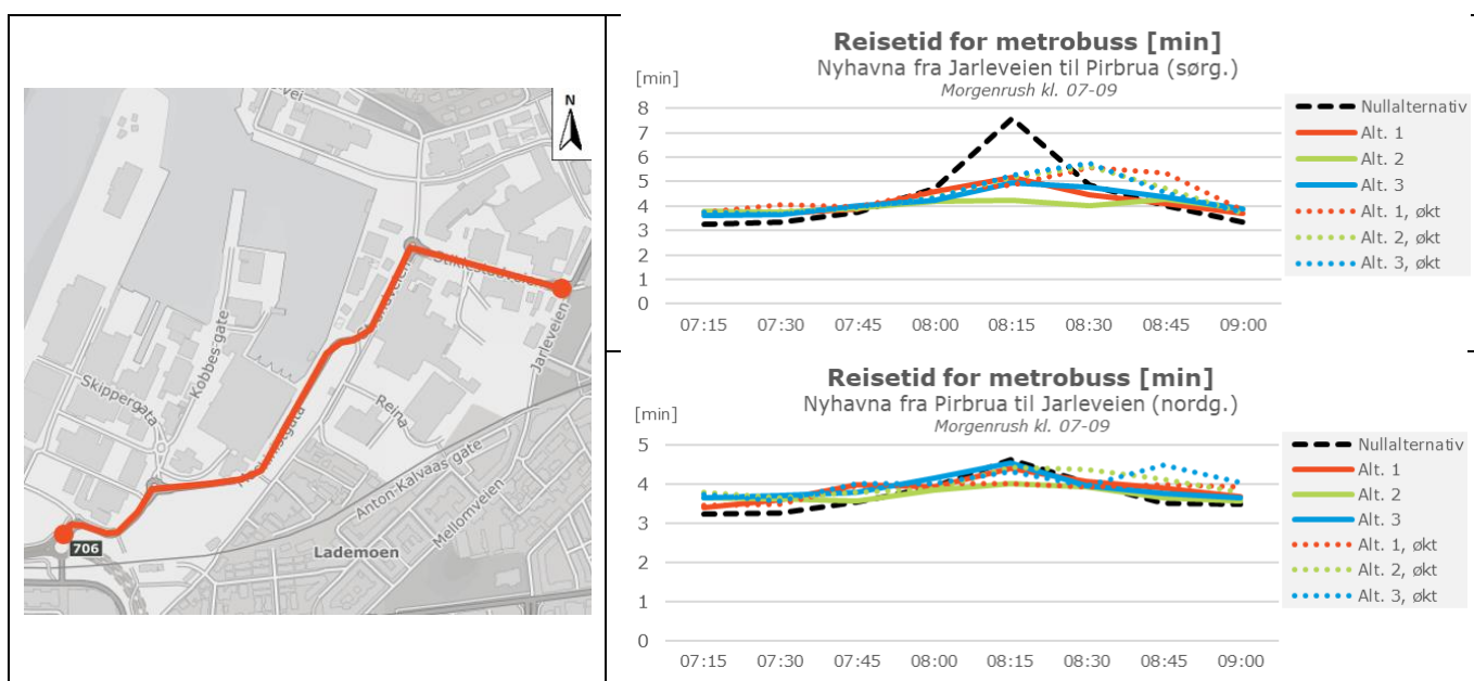
Figur 7-36: Reisetid for metrobusser gjennom Nyhavna, følsomhetsberegninger med økt trafikk, morgen
