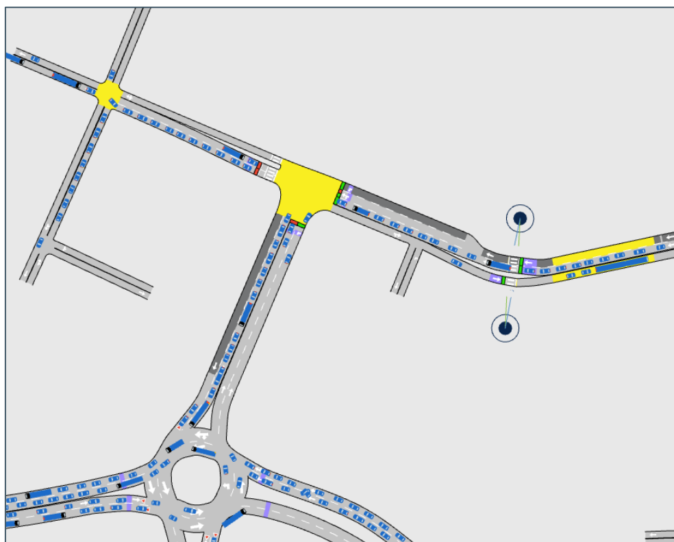
Figur 5-27: Simulering viser køoppbygging ut fra Båtmannsgata. Trafikk fra Båtmannsgata klarer ikke alltid å kjøre gjennom krysset med Skippergata
