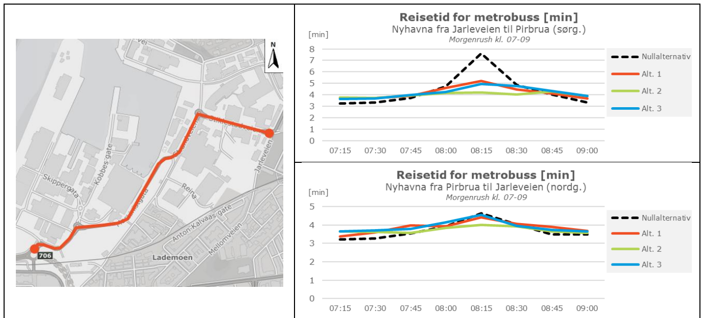
Figur 7-24: Reisetid for metrobusser gjennom Nyhavna, morgen
