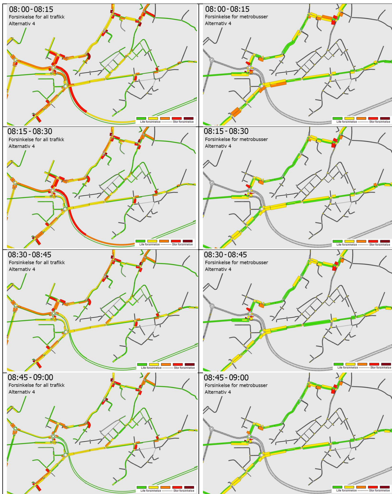
Figur 5-13: Forsinkelsesplot per kvarter i alternativ 4, morgen. All trafikk er vist til venstre og metrobuss til høyre.
