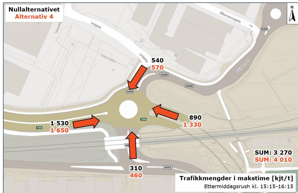
Figur 5-22: Sammenligning av avviket trafikk [kjt/t] nullalternativet og alternativ 4, i rundkjøring ved Strindheimtunnelen, ettermiddag
