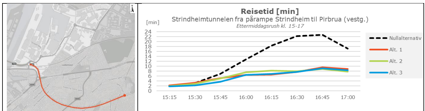
Figur 7-38: Reisetid i Strindheimtunnelen i vestgående retning, ettermiddag
