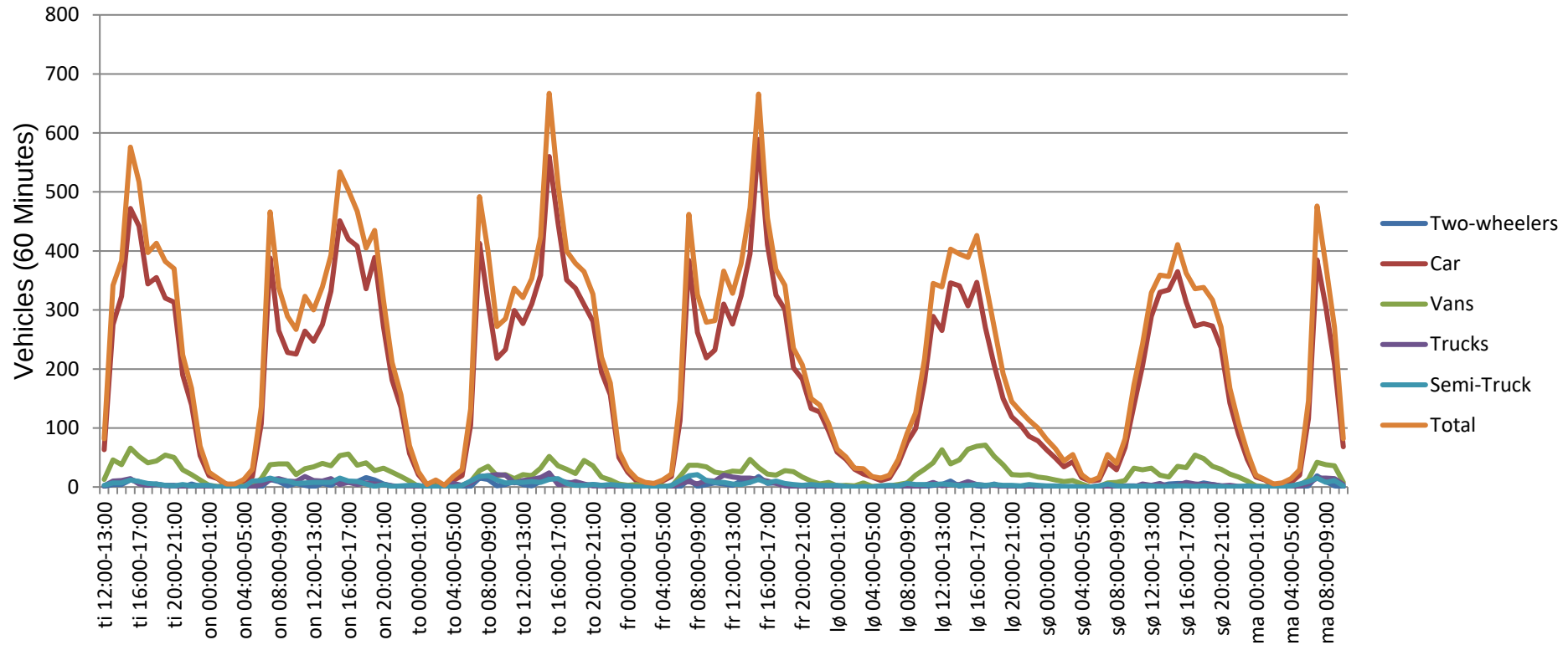
Figur 4: Trafikktelling tirsdag 23.januar – mandag 29.januar. Antall kjøretøy per time i Arnt Smistads veg. Kilde: Via traffic controlling
