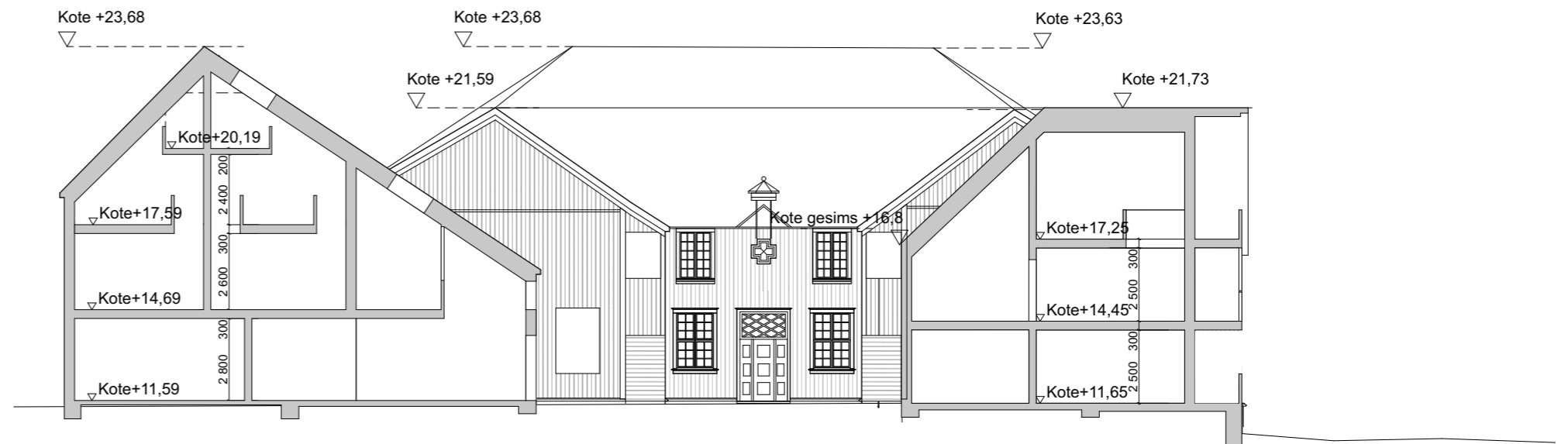
Snitt D-D
