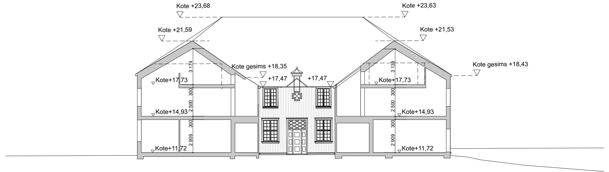
Snitt C-C
