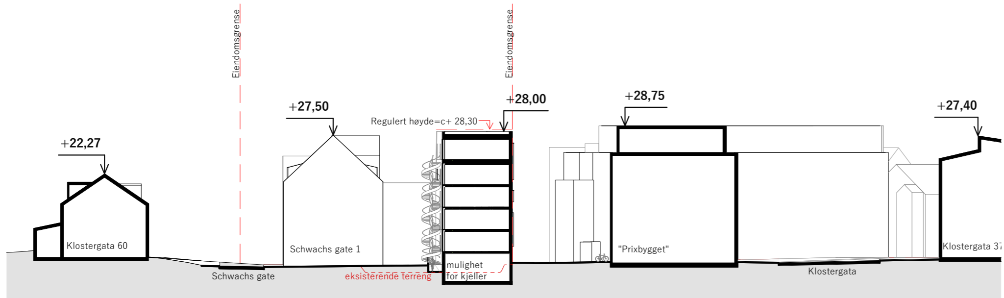
SITUASJONSSNITT A 1:500
