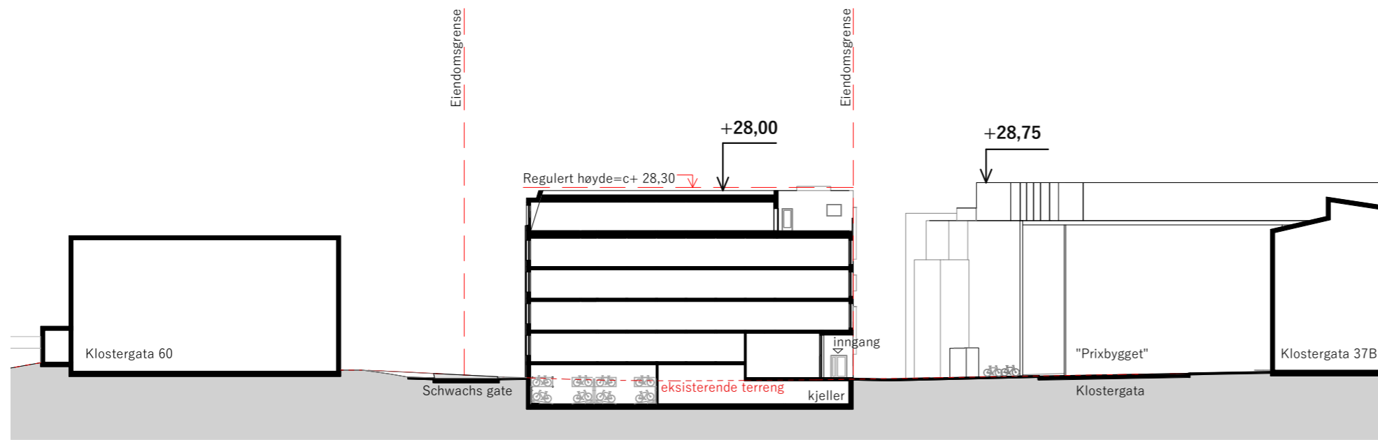
SITUASJONSSNITT B 1:500
