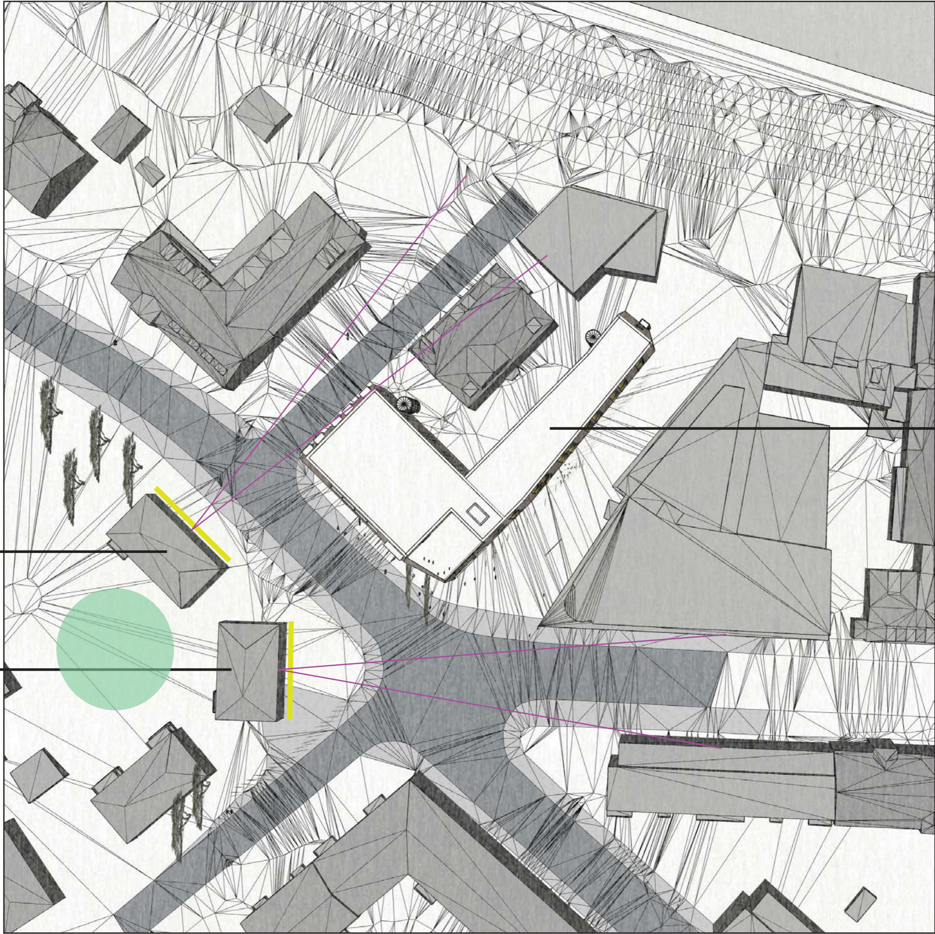
SITUASJONSPLAN
