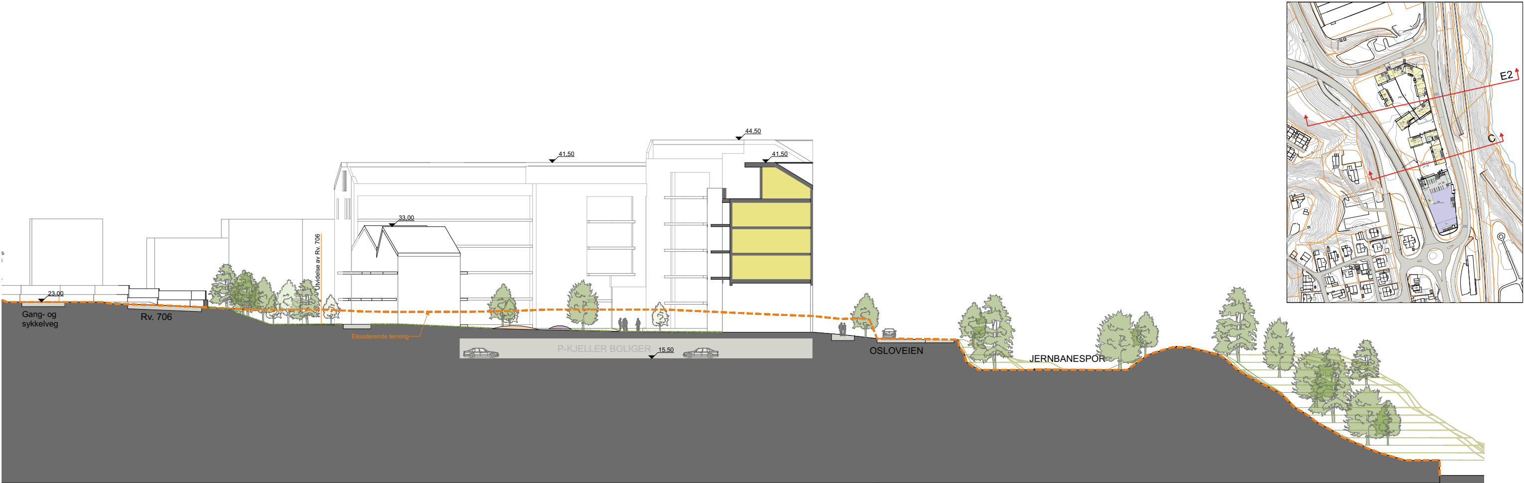
Snitt E2 1:500
