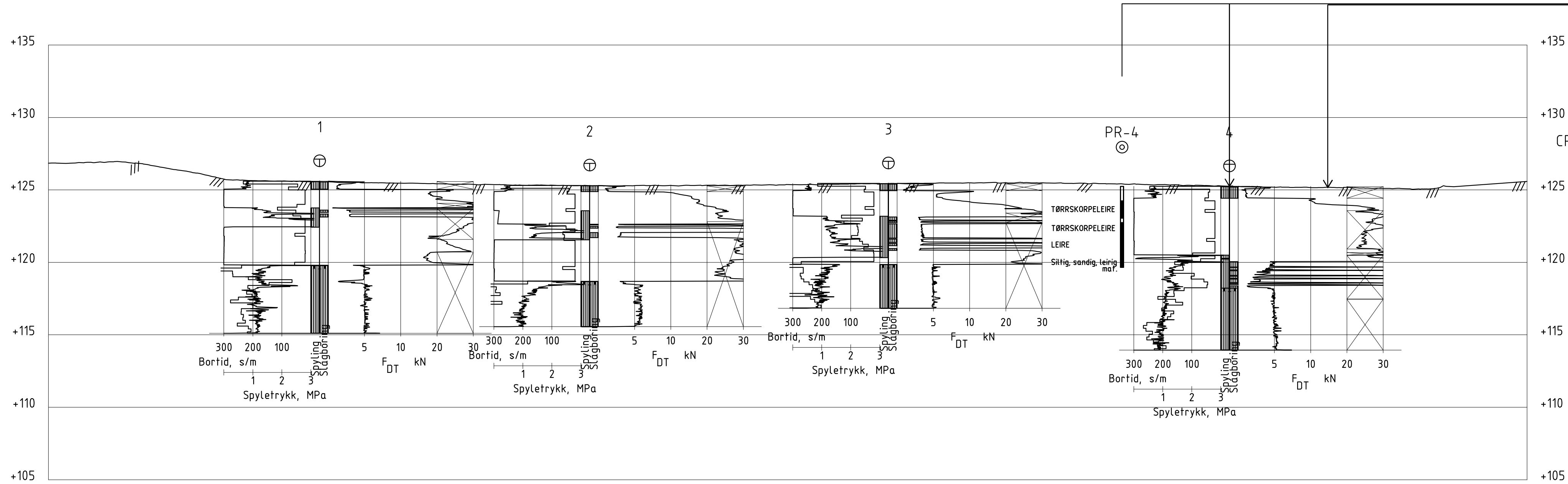
Profil A-A
