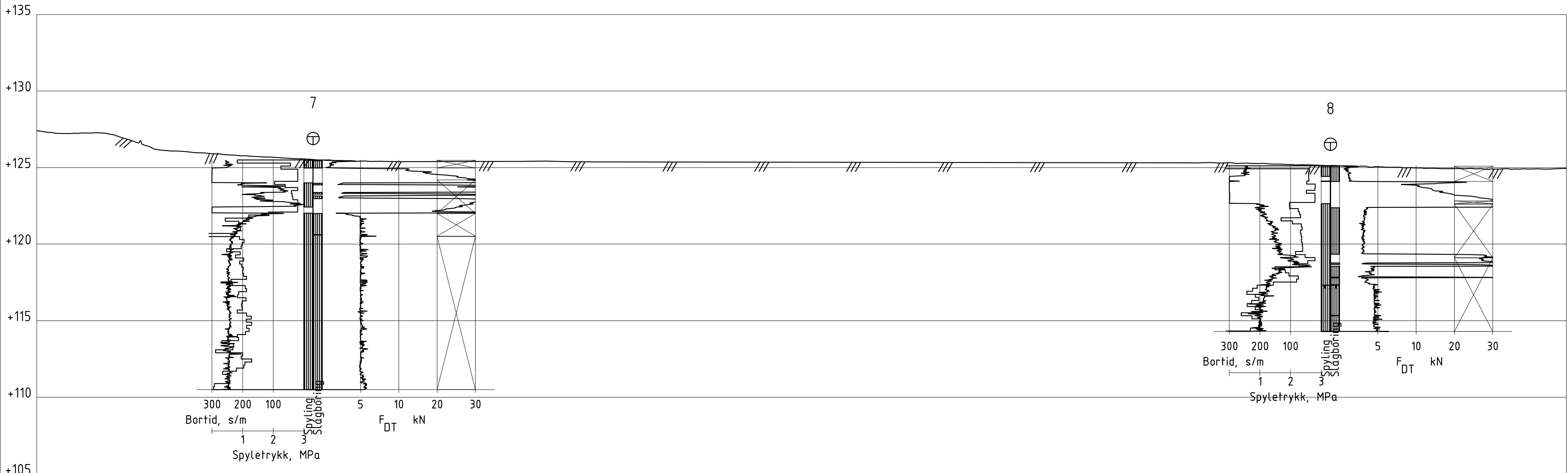
Profil C-C
