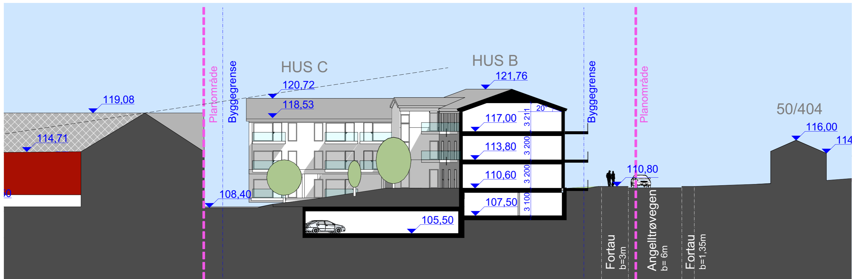
Snitt B
