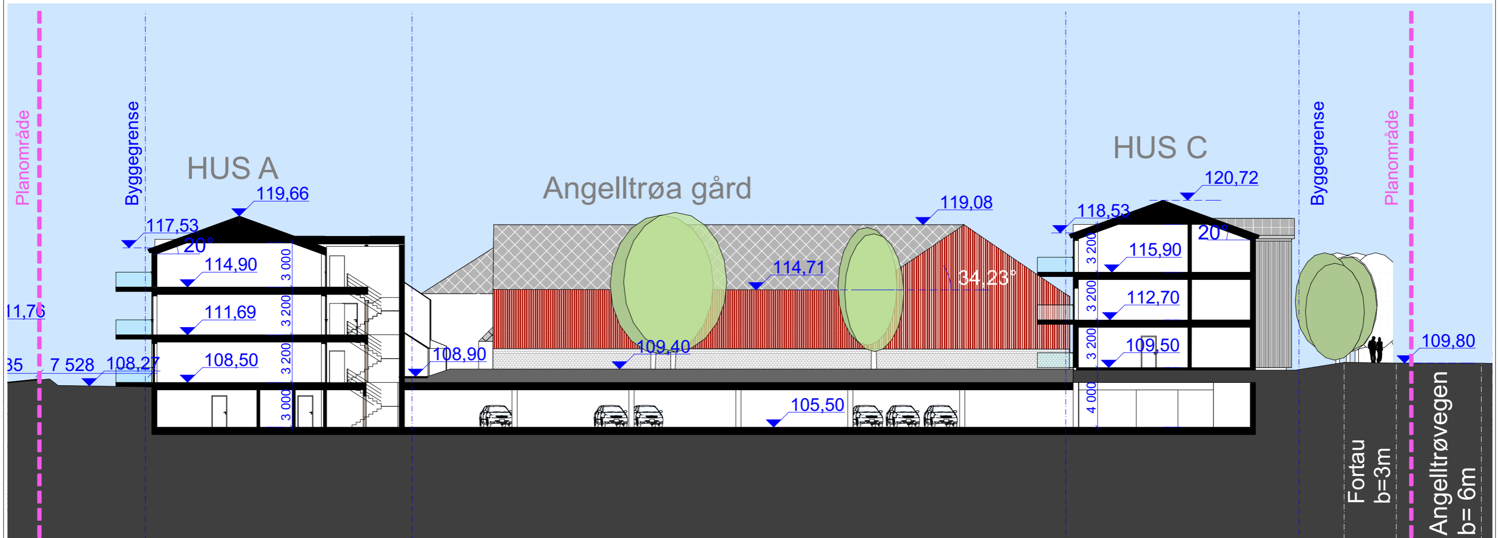
Snitt A
