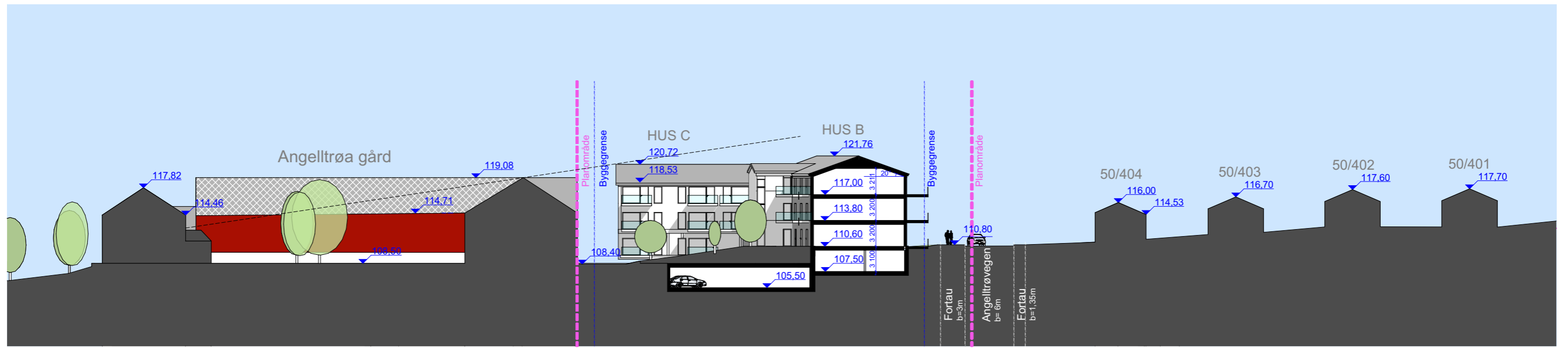
Snitt B
