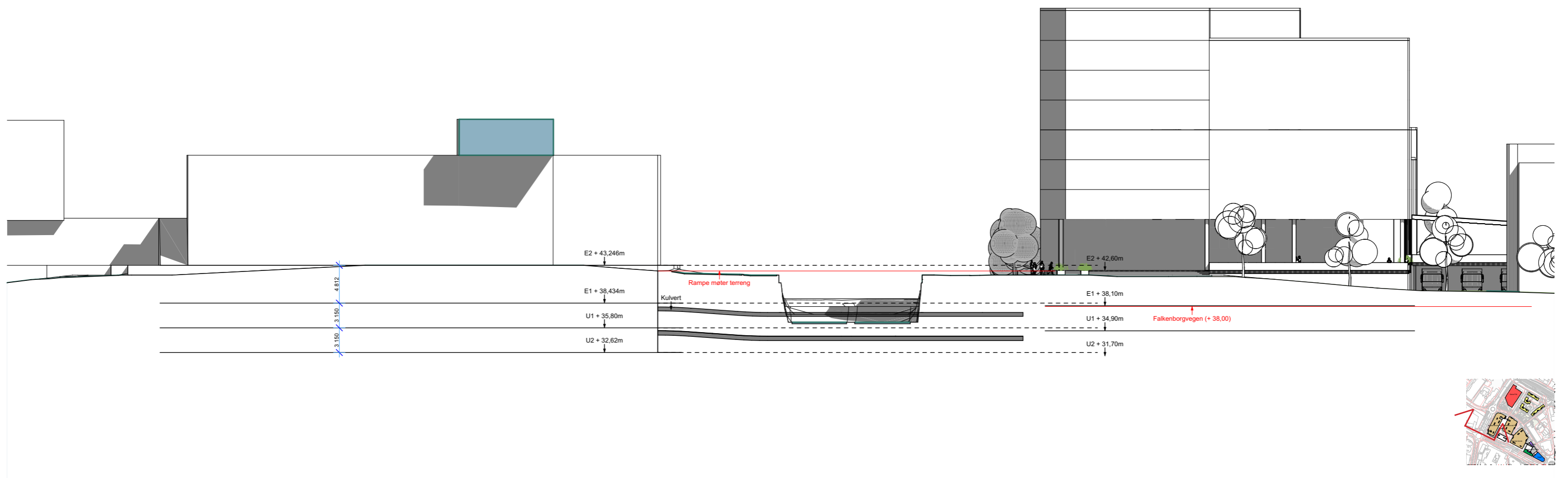
Snitt - Kulvert, mellom planområdet og sirkus Leangen sentrum - Illustrasjoner Alternativ 2
