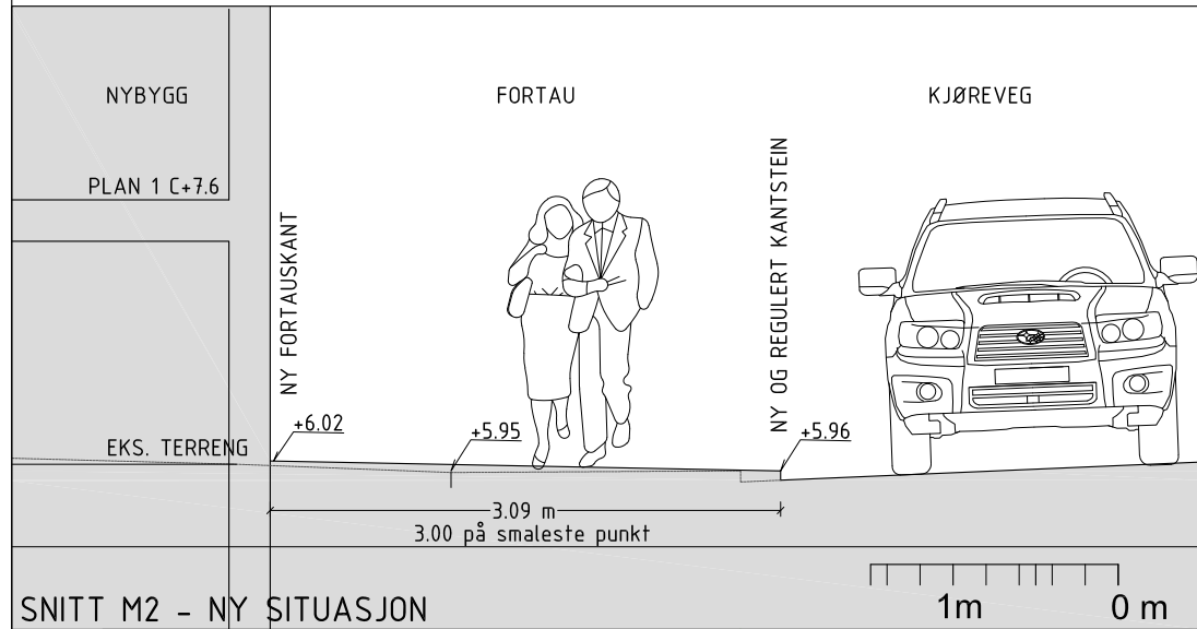
SNITT - M=1:50
