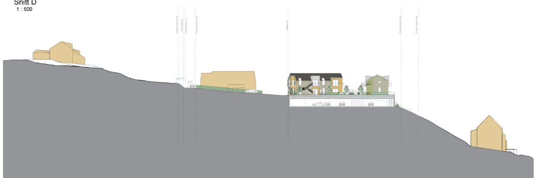
Snitt C 1 : 500
