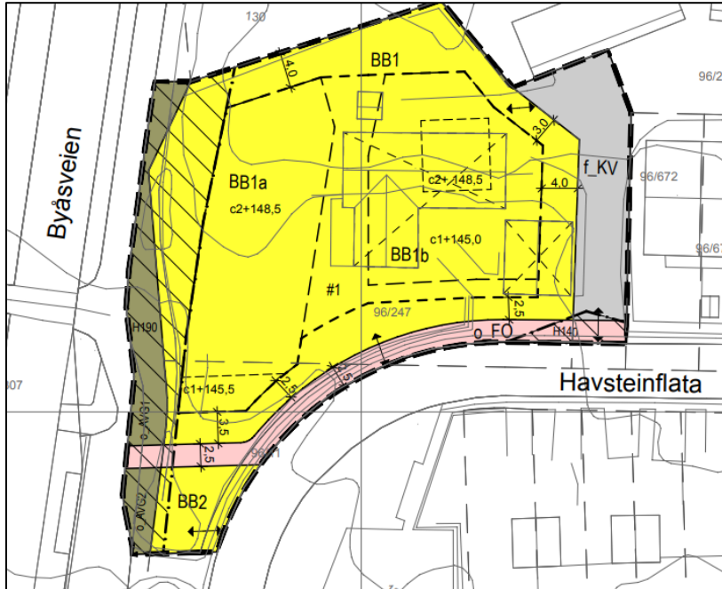
Figur 7: Plankart reguleringsplan Havsteinflata 7
