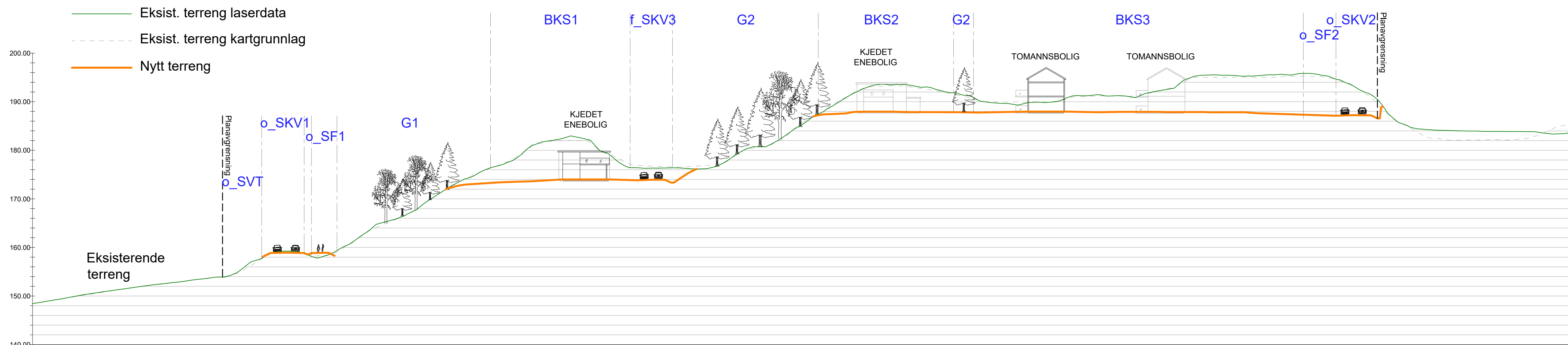
SNITT F
