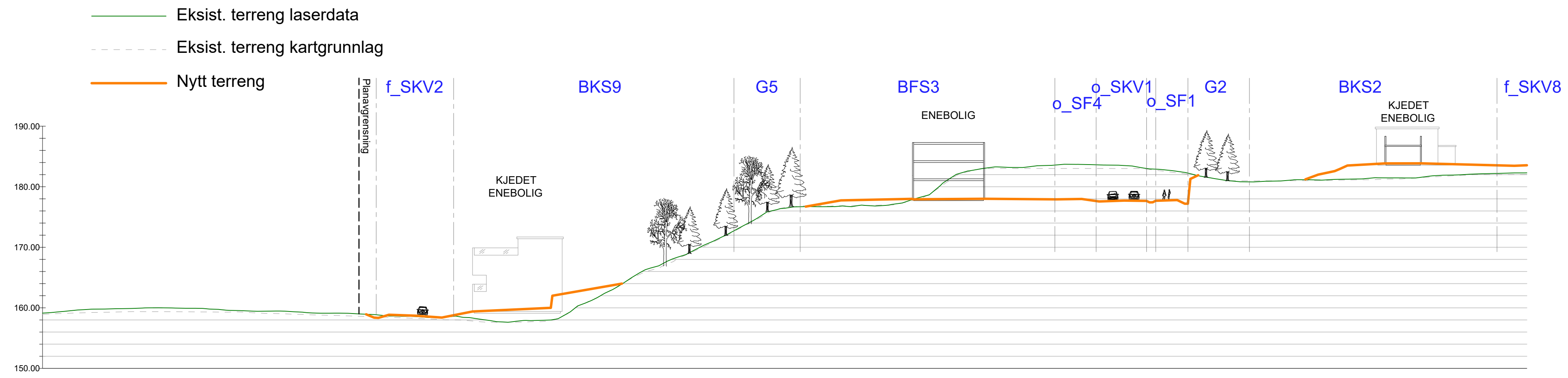
SNITT K
