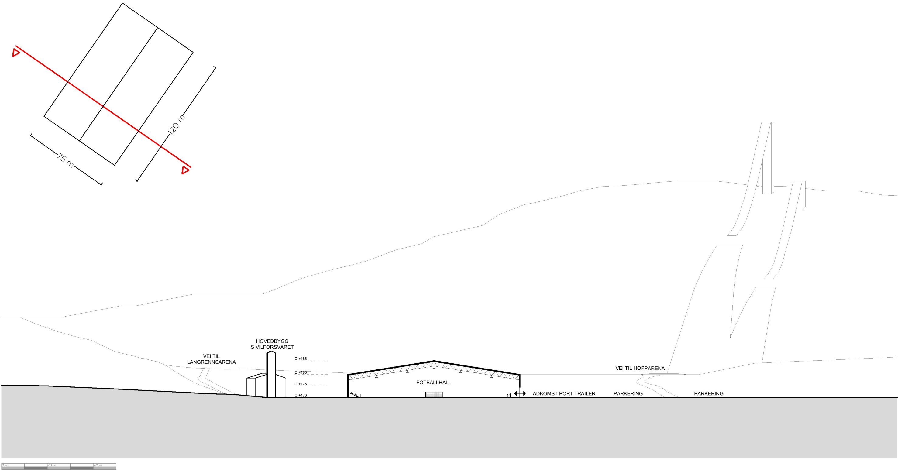
SNITT FOTBALLHALL 1:1000/A3
