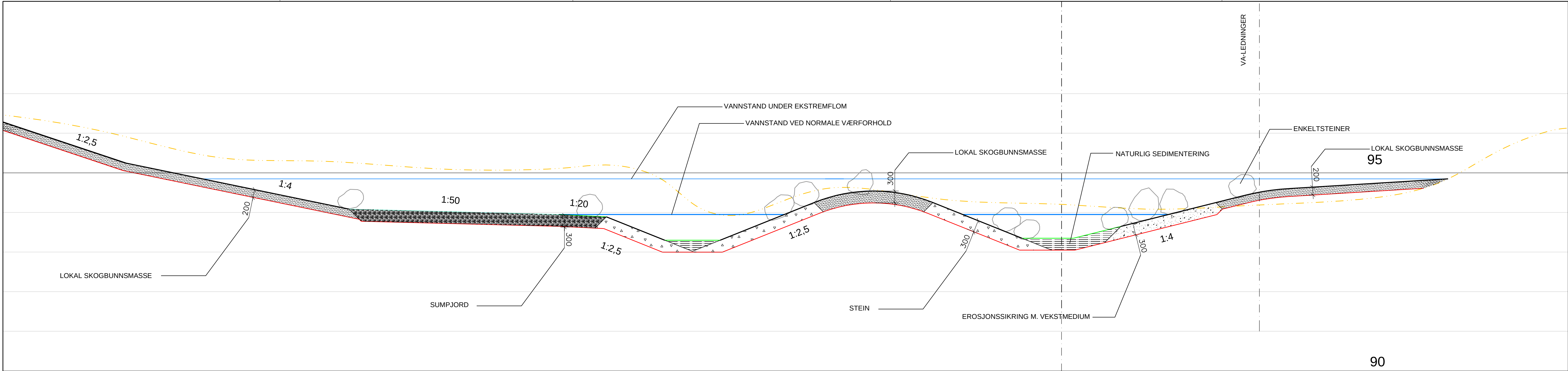
PROFIL 345 DAM 02 SETT MOTSTRØMS
