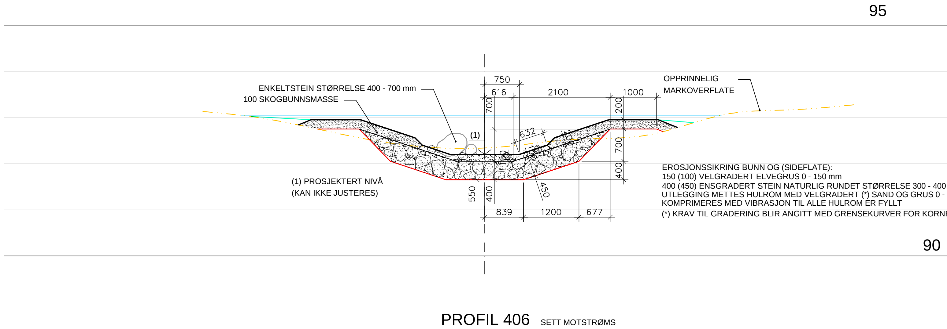
PROFIL 406 SETT MOTSTRØMS
