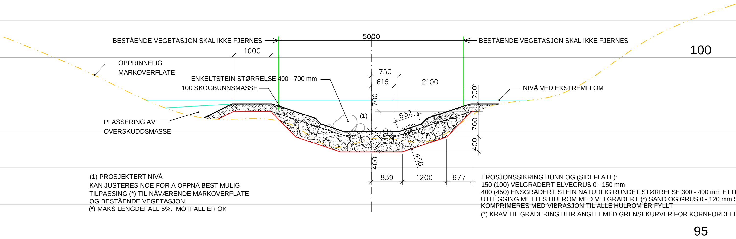
PROFIL 208 SETT MOTSTRØMS
