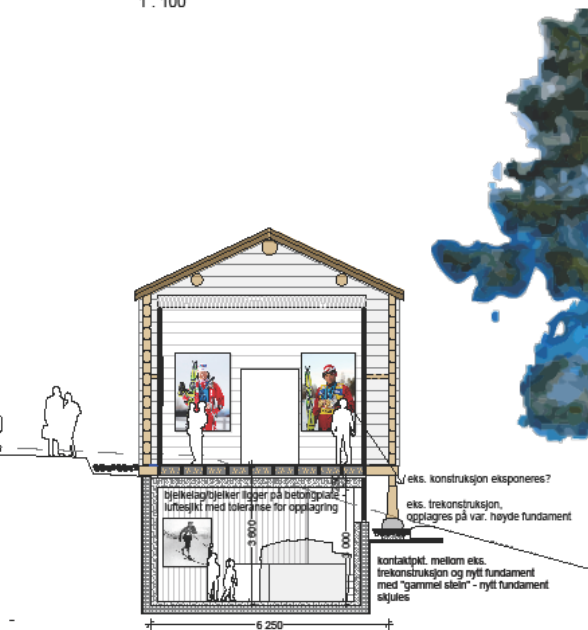
Snitt BB 1 : 100
