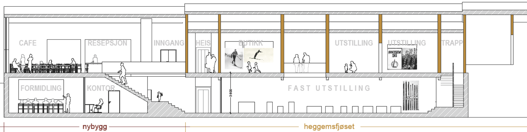
Langsnitt 1 : 100
