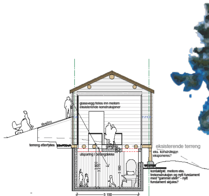
Snitt CC 1 : 100
